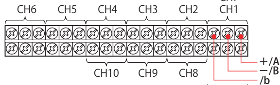
FX1010の 入力端子ブロック
