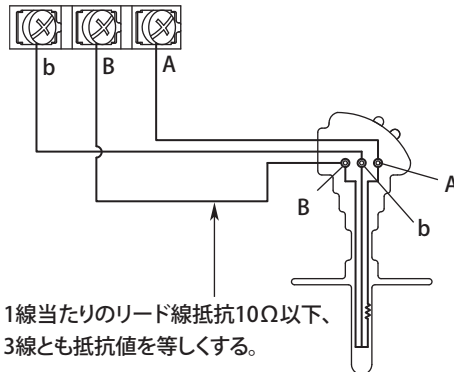
測温抵抗体入力
