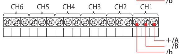
FX1006の 入力端子ブロック
