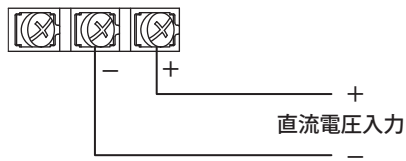
直流電圧入力およびDI(ON/OFF)入力
