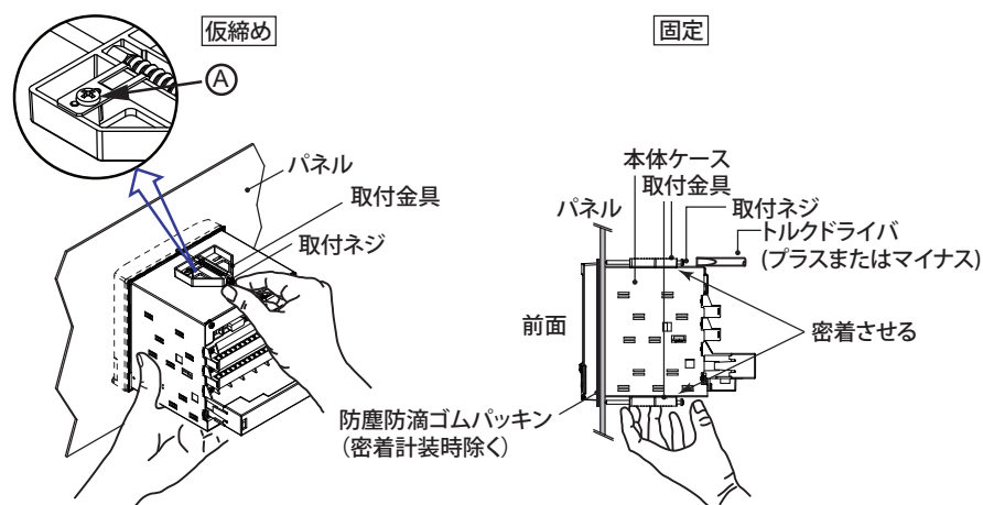
パネル取り付け図
