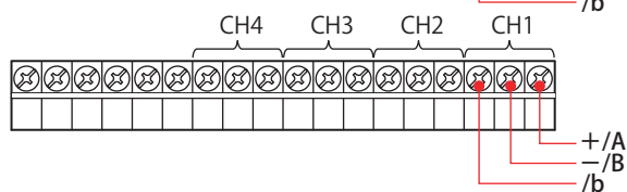
FX1004の 入力端子ブロック
