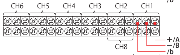
FX1008の 入力端子ブロック
