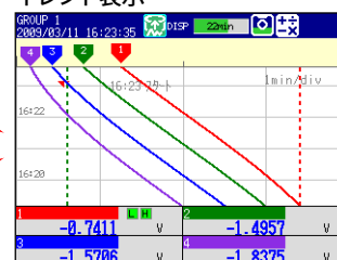
トレンド表示
