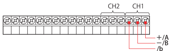
FX1002の 入力端子ブロック
