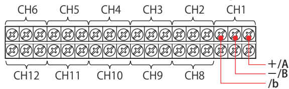
FX1012の 入力端子ブロック
