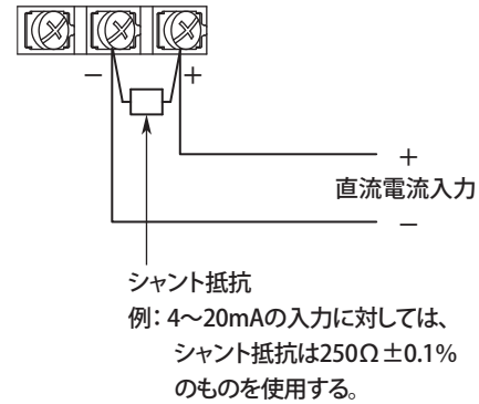
直流電流入力
