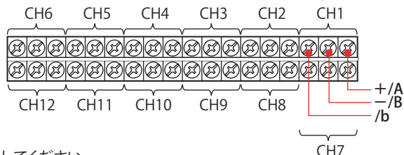
FX1012の 入力端子ブロック
