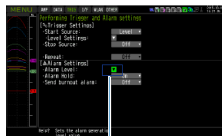
警報條件設定
